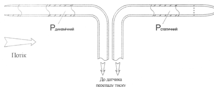
Рис. 1. Приклад конструкції напірної трубки
