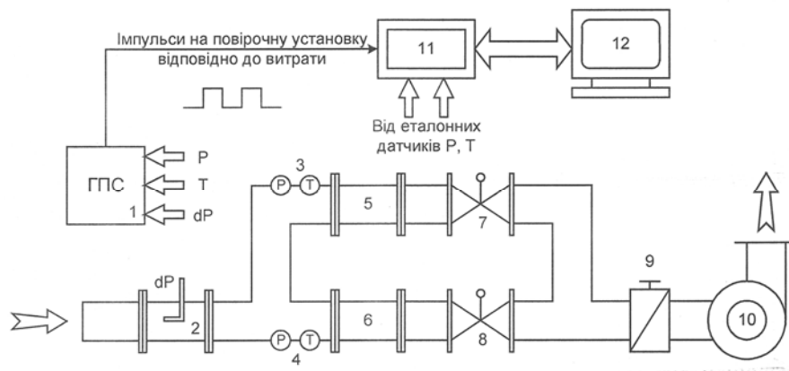
Рис. 2. Схема під'єднання ГПС до установки УПЛГ-2500:
